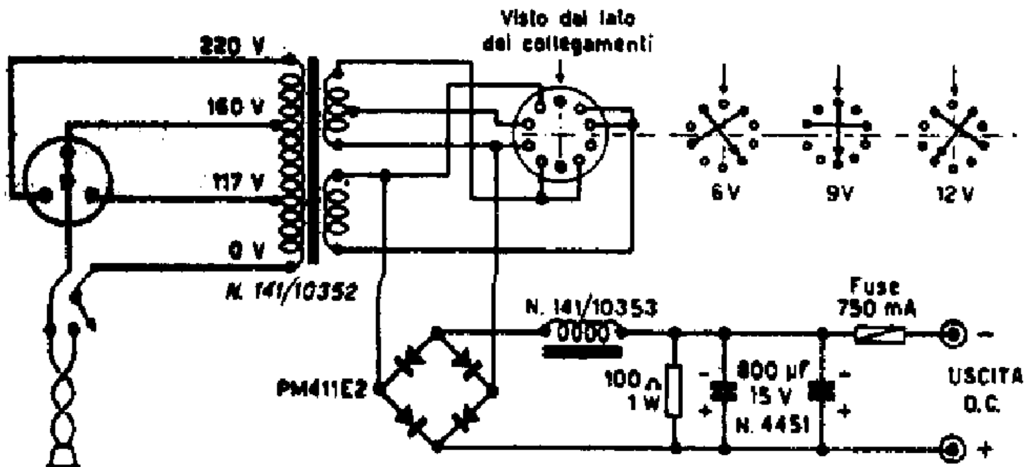
Alimentatore N° 1489
